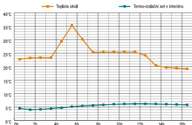
Teplotní křivka v termo-izolačním setu Léto
