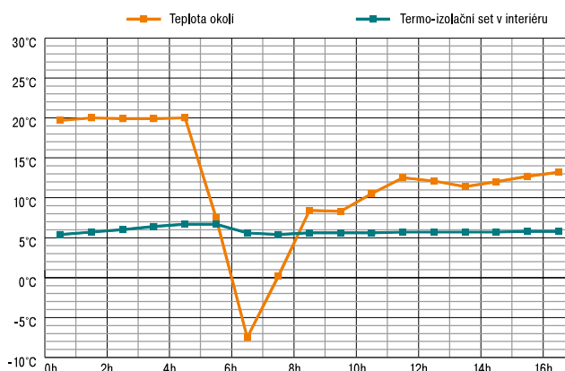
Teplotní křivka v termo-izolačním setu Zima
